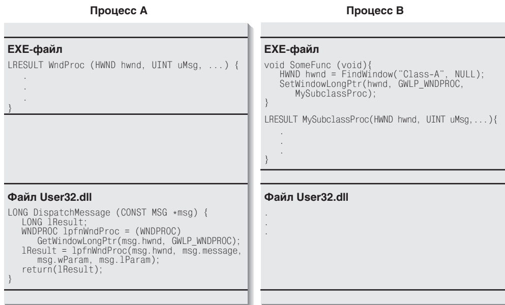
Рис. 22-1. Поток процесса В пытается создать подкласс окна, сформированного потоком процесса А
