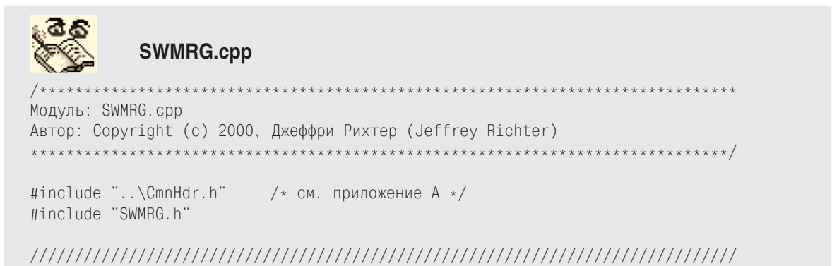
Рис. 10-3. Программа-пример SWMRG
