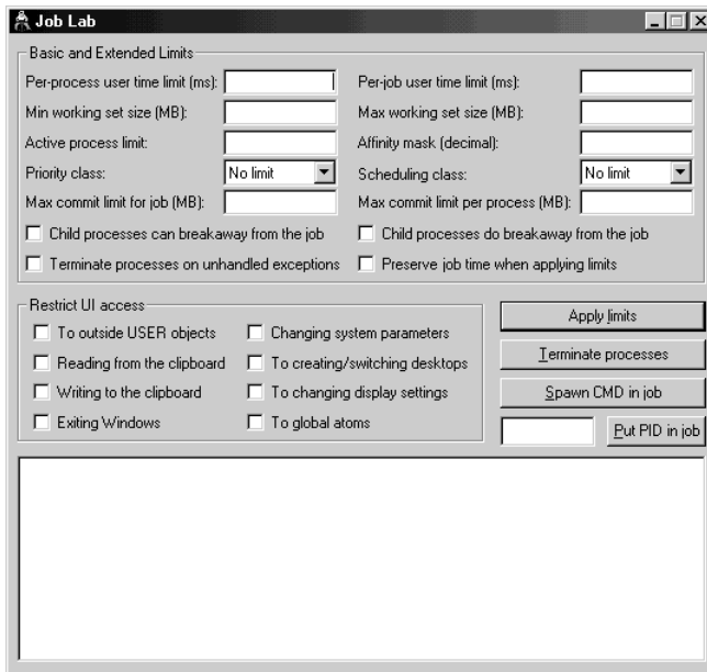
Рис. 5-5. Программа-пример JobLab
