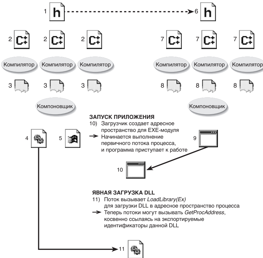
Рис. 20-1. Так DLL создается и явно связывается с приложением
