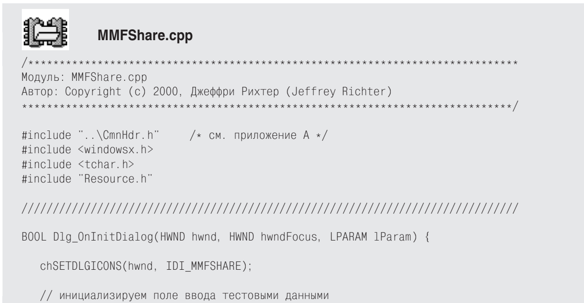
Рис. 17-3. Программа-пример MMFShare
