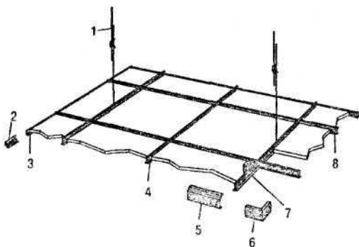
Рис. 1. Схема сборки подвесного потолка
